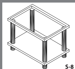
S-8
