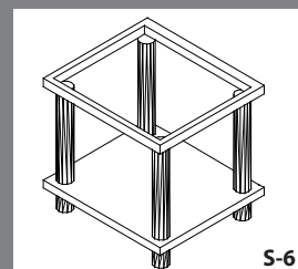
S-6
