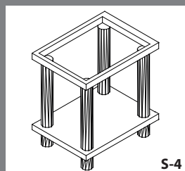
S-4
